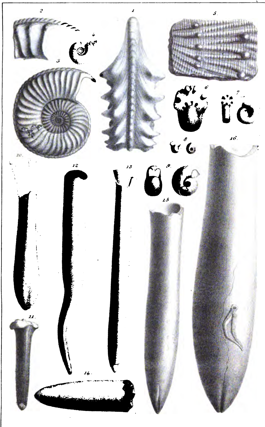
Siemstady, Jura.
